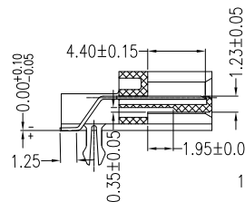
SECT A-A
