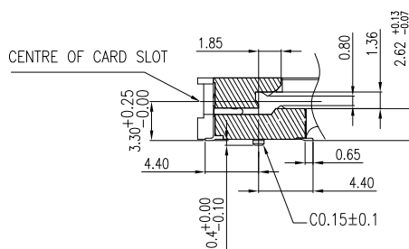
SECTION:A-A SCALE 2:1
