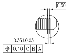
DETAIL:C SCALE 2:1
